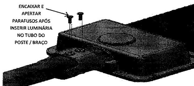
Sistema de fixação em poste / braço reto
