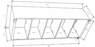
Perspectiva Caixa Armário Fig. 1.20
