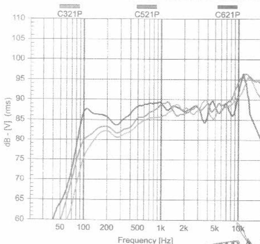
Curva de resposta em câmara anecóica, 1W@1m.
