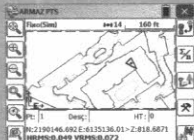
Armazenar Pontos em Modo Gráfico.
